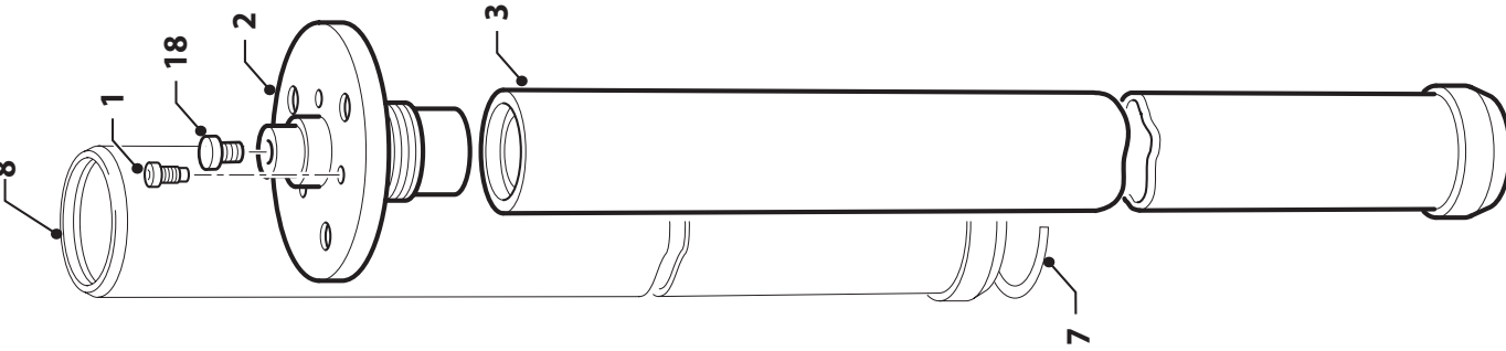
NAJMNIEJSZA RURA Z PŁYTĄ MONTOWANĄ A 3 ŚRUBY
