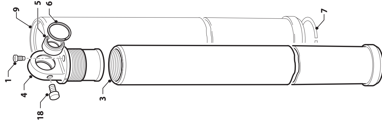
NAJMNIEJSZA RURA Z DEMONTOWALNYM UCHEM
